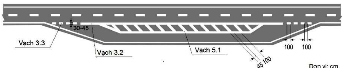
Hình G.19 - Bố trí vạch ở điểm dừng xe kiểu bến cảng, trường hợp sử dụng vạch 5.1
