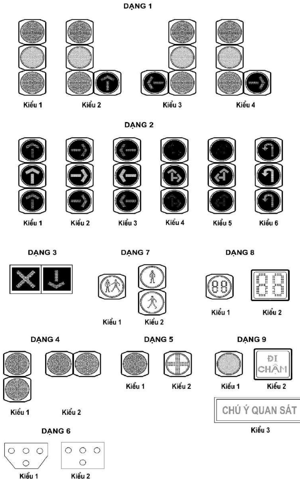
Hình A.1. Các dạng đèn tín hiệu
