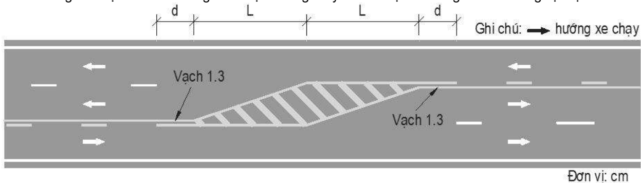
Ghi chú: Khoảng cách d = 75 m, khoảng cách L \geq 25 m. Hình G.8 - Bố trí vạch sơn phân chia hai chiều xe chạy cho đường có 3 làn xe trong khu vực số làn trên một hướng thay đổi từ một làn sang hai làn
