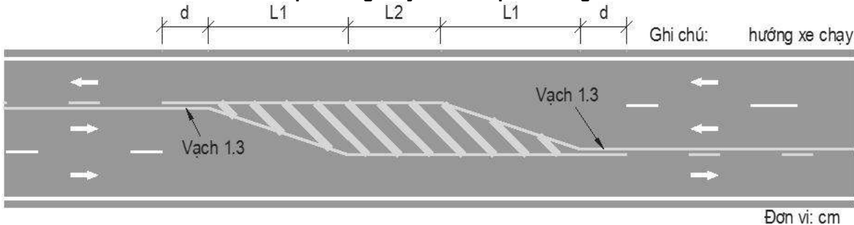
Ghi chú: Khoảng cách d = 75 m, L1 \geq 100 m, khoảng cách L2 \geq 100 m. Hình G.9 - Bố trí vạch sơn phân chia hai chiều xe chạy cho đường có 3 làn xe trong khu vực số làn trên một hướng thay đổi từ hai làn sang một làn
